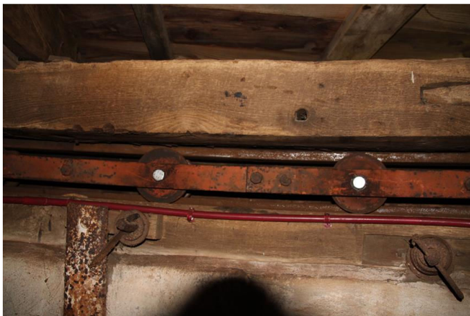
Rollenwerk hersteld, en kruiring rond gericht.
