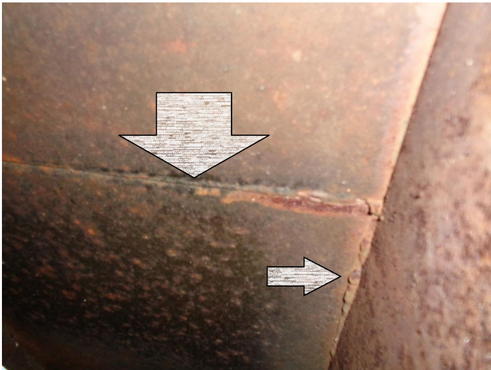
Slecht door gelaste lassen Derkx roede na opname uitgeslepen en doorgelast.
